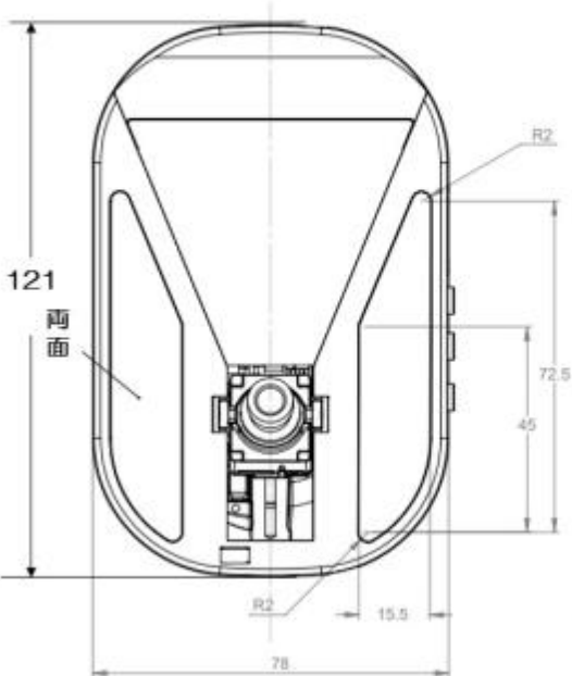
本体図（ガラス貼付け面）
